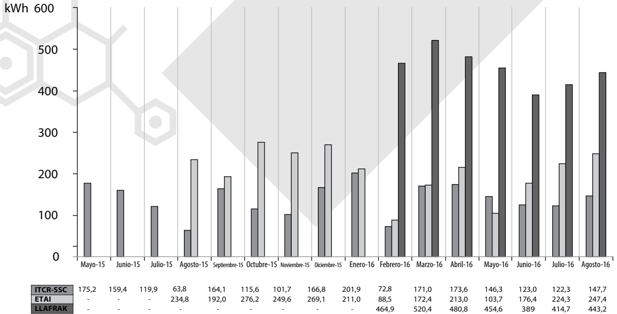
FIGURA 38. COMPARATIVA DE LA ENERGÍA CALORÍFICA MENSUAL PRODUCIDA POR LOS SISTEMAS TÉRMICOS DE CALENTAMIENTO DE AGUA, EN LAS LECHERÍAS DEL ITCR-SSC Y ETAI Y EN LA PLANTA PROCESADORA DE LÁCTEOS LLAFRAK DE JUANILAMA DE POCOSOL.
