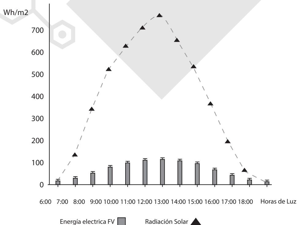
FIGURA 37. ENERGÍA SOLAR Y ENERGÍA ELÉCTRICA GENERADA POR DÍA (PROMEDIO ANUAL).
