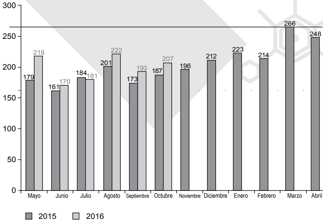
FIGURA 35: ENERGÍA TOTAL GENERADA MENSUALMENTE POR EL SISTEMA FOTOVOLTAICO DURANTE EL AÑO Y MEDIO DE ESTUDIO EN LA LECHERÍA DEL ITCR-SSC.
