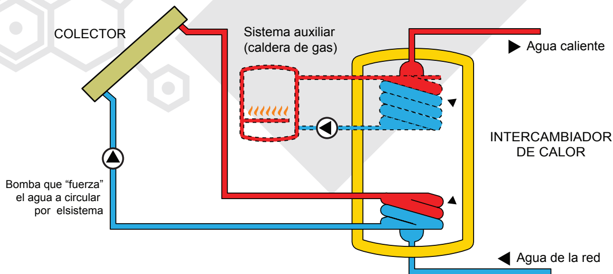
FIGURA 8. FUNCIONAMIENTO BÁSICO DE UN COLECTOR TÉRMICO-HÍBRIDO FORZADO.
