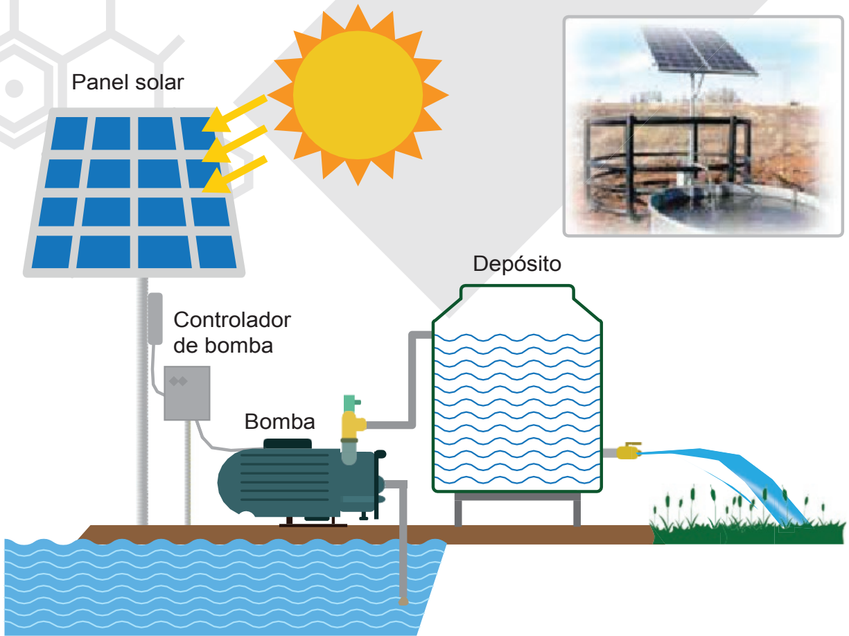
FIGURA 19. BOMBA SOLAR PARA EXTRACCIÓN DE AGUA DE UN POZO.
