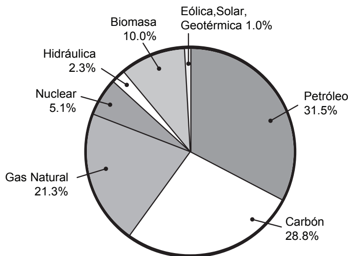
FIGURA.1: CONSUMO MUNDIAL DE FUENTES DE ENERGÍA. (FUENTE: AIE, 2016).
