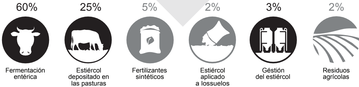
FIGURA 3. PRINCIPALES EMISORES DE GASES DE EFECTO INVERNADERO A LA ATMÓSFERA DENTRO DE LA GANADERÍA. (IMAGEN: MODIFICADO DE LIRA, J. (2014).)
