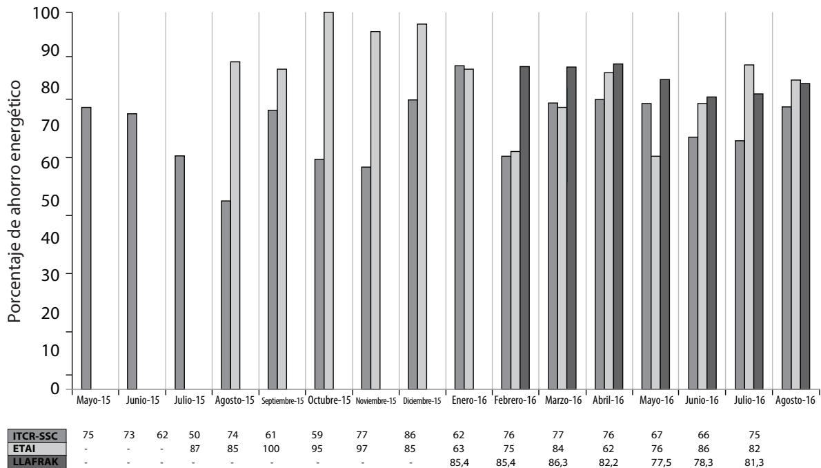
FIGURA 39. COMPARATIVA DEL AHORRO ENERGÉTICO DE LOS SISTEMAS TÉRMICOS EN LAS DIFERENTES INSTALACIONES.
