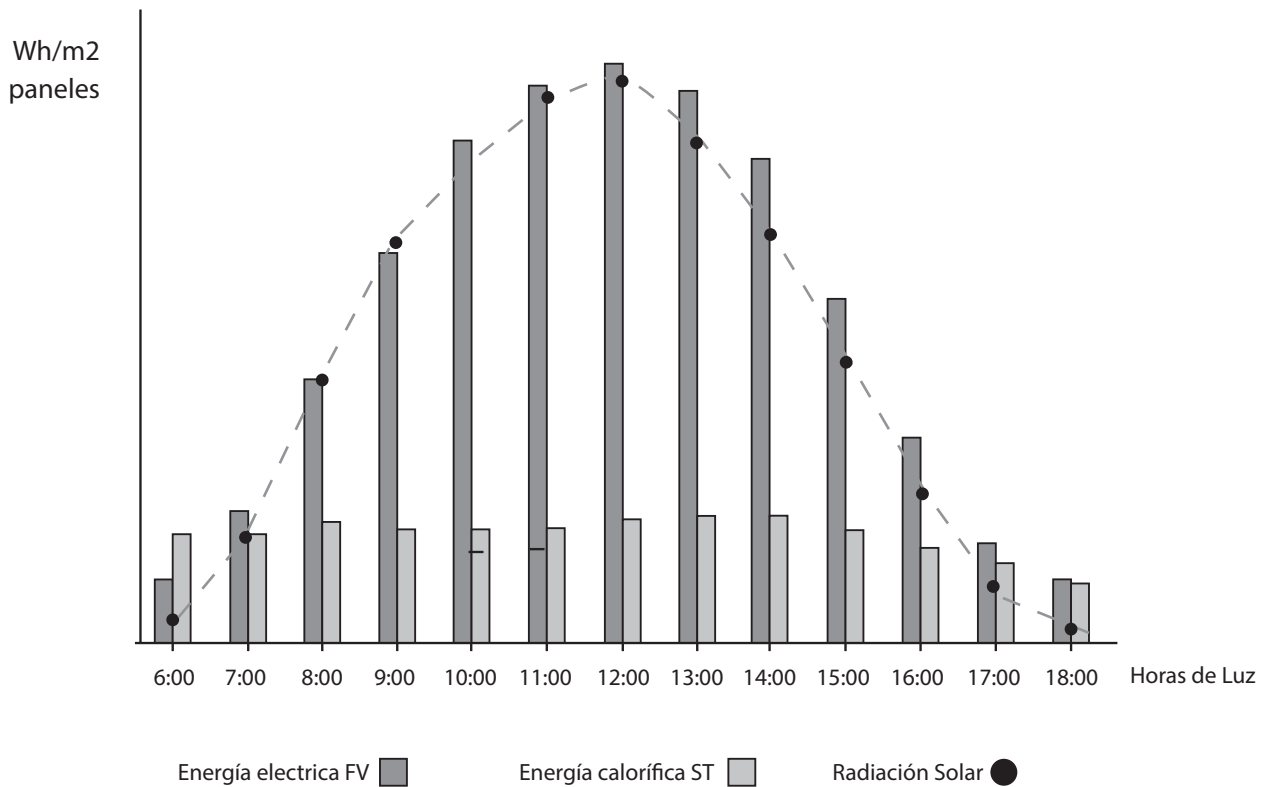
FIGURA 41. PRODUCCIÓN ENERGÉTICA DE LOS PANELES FOTOVOLTAICOS Y TÉRMICOS A LO LARGO DE UN DÍA DE LUZ (EN WH POR M 2 ) EN LA LECHERÍA DEL ITCR-SSC.
