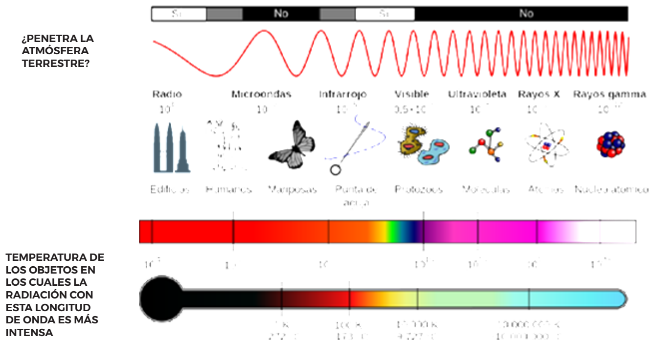
FIGURA 5. ESPECTRO ELECTROMAGNÉTICO.
