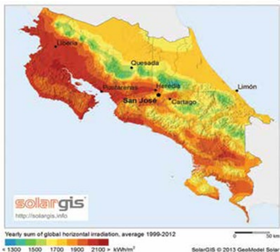
FIGURA 11. RADIACIÓN GLOBAL RECIBIDA EN COSTA RICA.
